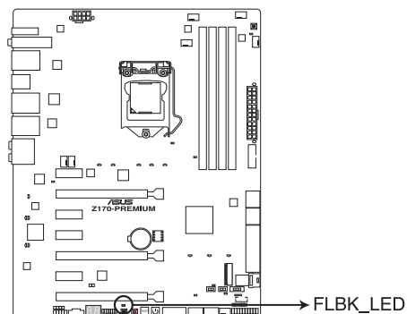
Z170-PRIME FLBK_LED
