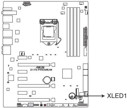
Z170-PRIME XLED1
