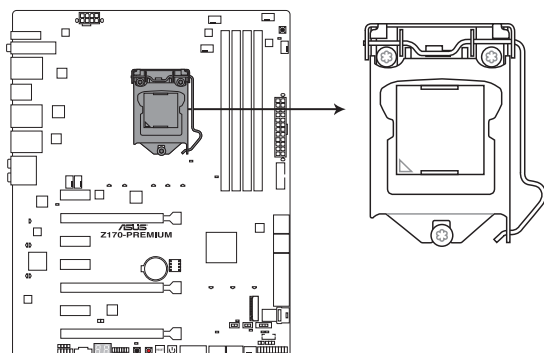
Z170-PRIME CPU LGA1151
