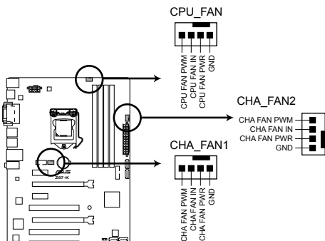
Z87-K Fan connectors
