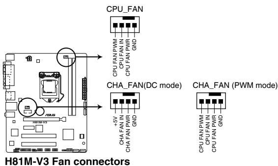
H81M-V3 Fan connectors
