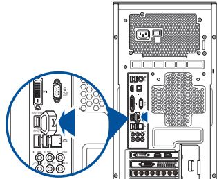
後面板
